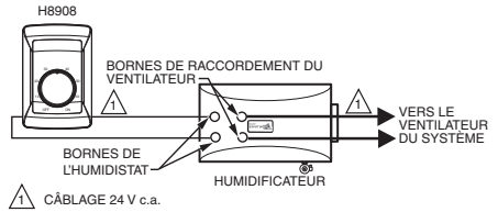
Fig. 16. Raccordement du H8908 avec un humidificateur à vapeur.
