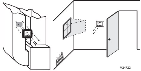
Fig. 9. Poser la plaque de montage sur la gaine ou sur le mur.
