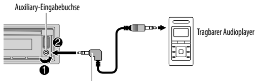
3,5-mm-Stereo-Ministecker mit "L"-förmigem Anschluss (im Handel erhältlich)
