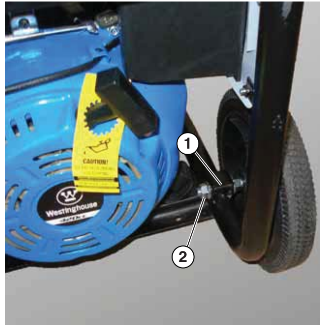
Figura 9 – Ensamble las ruedas al bastidor
