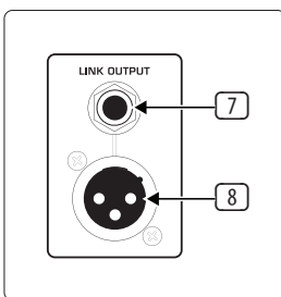
Fig. 2.4: LINK OUTPUT
