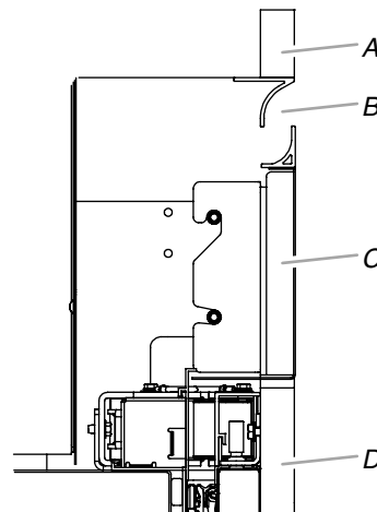
A. Soffite
