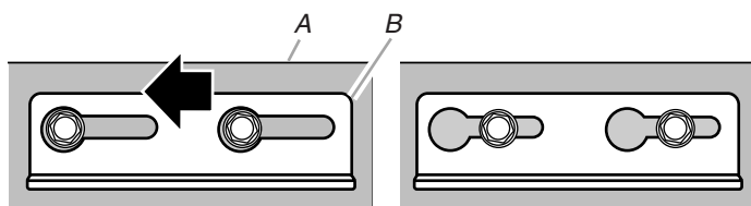
A. Door panel B. Panel top bracket
