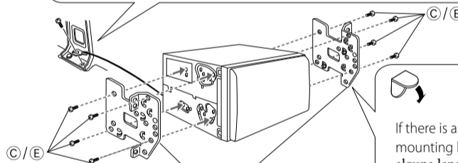
Mounting bracket removed from the car / Soporte de montaje removido del automóvil / Support de montage retiré de la voiture
