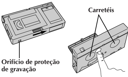
Fita de vídeo compacta
