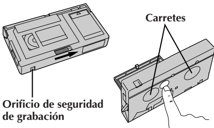
Cassette compacto VHS
