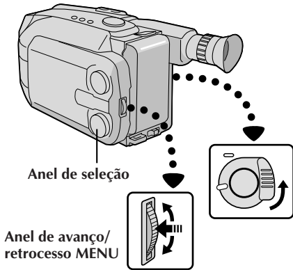
Monitor LCD ou visor eletrônico
