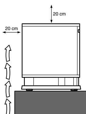
Zijaanzicht
