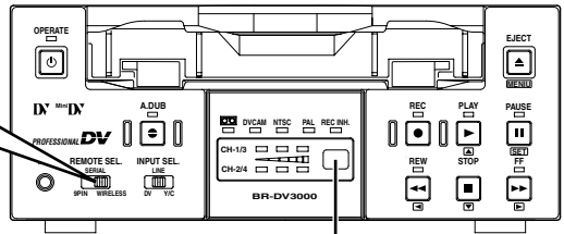
Sensor del mando a distancia inalámbrico
