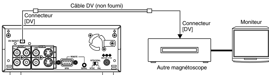
Lecteur : panneau arrière du magnéscope
