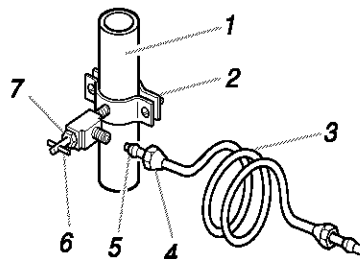
1. Canalisation d'eau froide 2. Bride de tuyau 3. Tube en cuivre 4. Écrou de compression 5. Bague de compression 6. Robinet d'arrêt 7. Écrou de serrage
