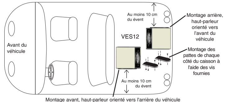
Montage avant, haut-parleur orienté vers l'arrière du véhicule
