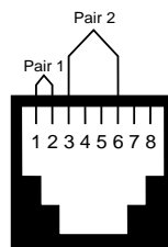
10BASE-T
