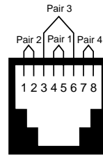
T568B
