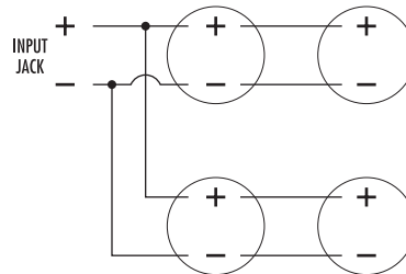
4 Ohm Wiring Setup
