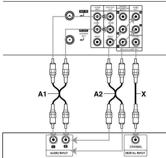
Amplificador (Receptor)
