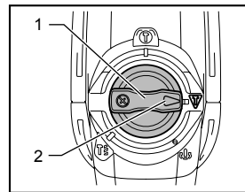
1. Levier de changement 2. Index
