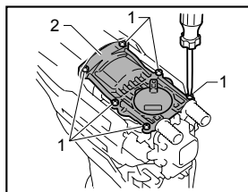
1. Vis 2. Capuchon de manivelle
