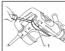
1. Protecteur
