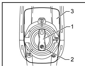
1. Levier de changement de mode 2. Vis 3. Couvercle du capuchon de manivelle
