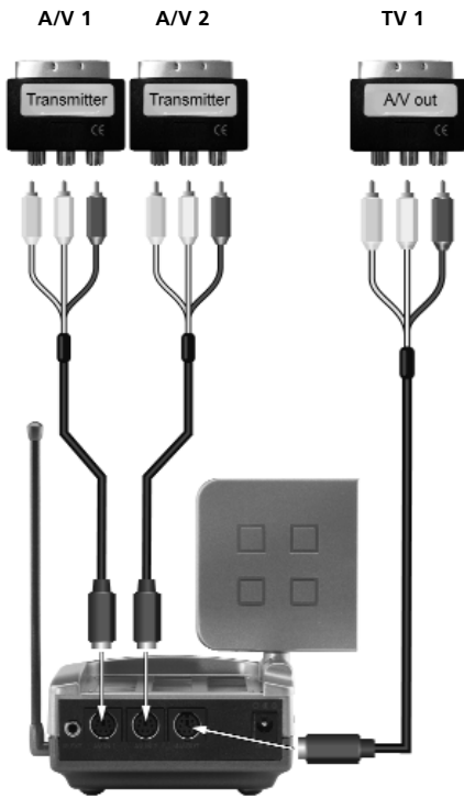
Afbeelding 1 A/V ZENDER
