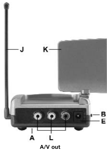
Afbeelding 4 A/V ONTVANGER
