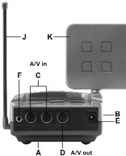
Abbildung 3 A/V SENDER
