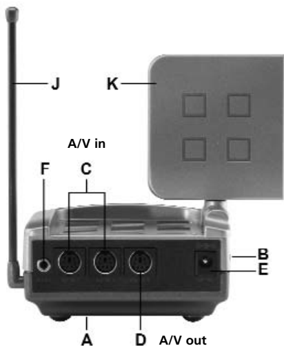
Figura 3 EMISOR A/V
