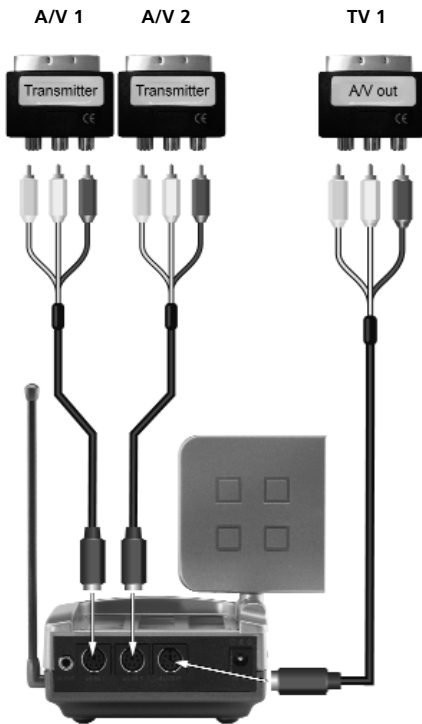
Abbildung 1 A/V SENDER
