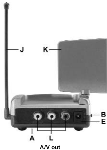
Immagine 4 RICEVITORE A/V
