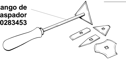
Raspador con hojas intercambiables
