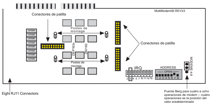
Figura 2-2. Componentes del módulo auxiliar y MultiModemISI
