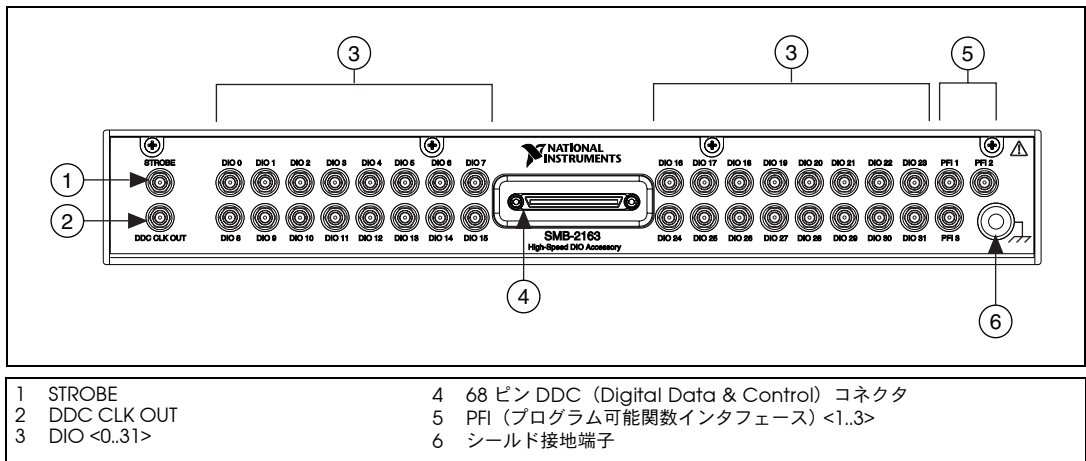
図 1 NI SMB-2163 パーツ配置図
