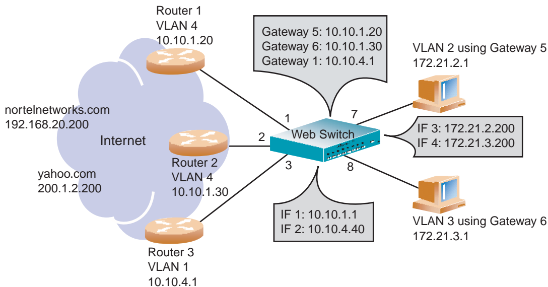
Figure 2-6 Default Gateways per VLAN
