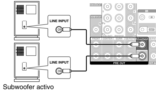
Subwoofer activo
