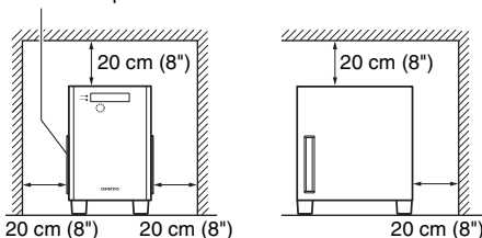
Bass-reflex port
