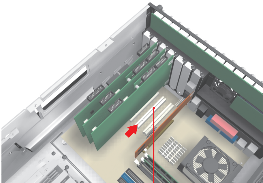
PCI SLOT2
