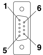
CN-2 (D-Sub 9-pin side)
