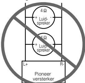
2 Ω brugschakeling
