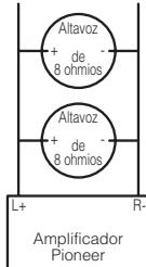
Modo de conexión en puente de 4 ohmios
