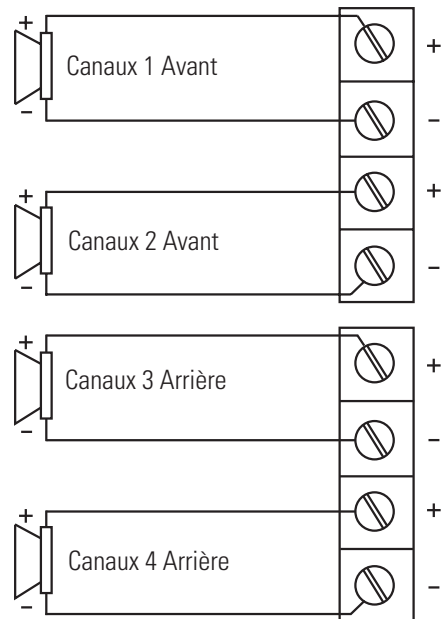
FIGURE 4—DIAGRAMMES DE CONNEXION DES HAUT-PARLEURS (PA1100.5)
