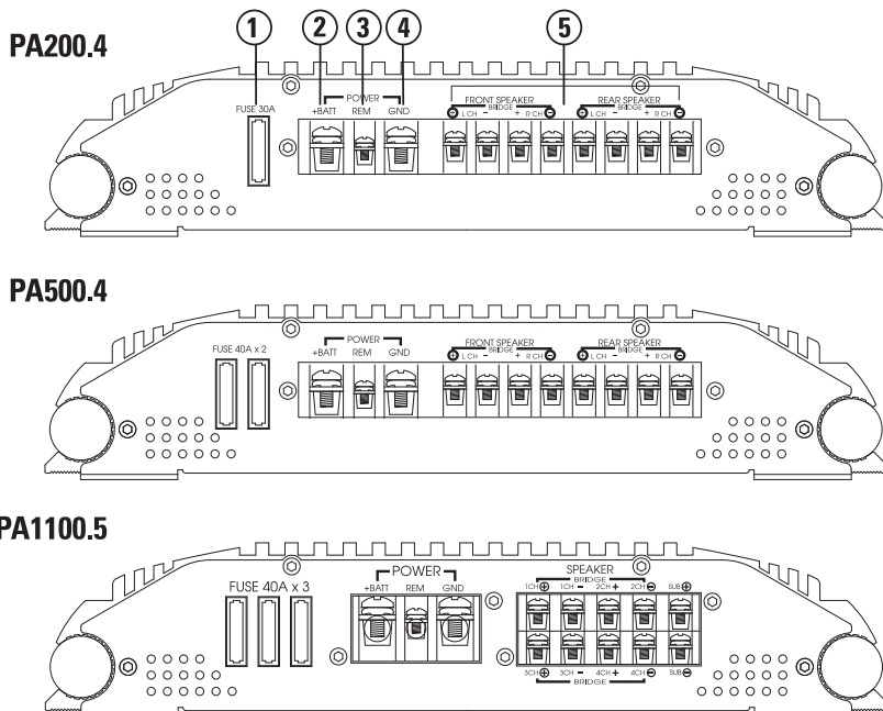
FIGURA 3—CONNESSIONI DELL'AMPLIFICATORE—LATO POSTERIORE (PA200.4/PA500.4/PA1100.5)
