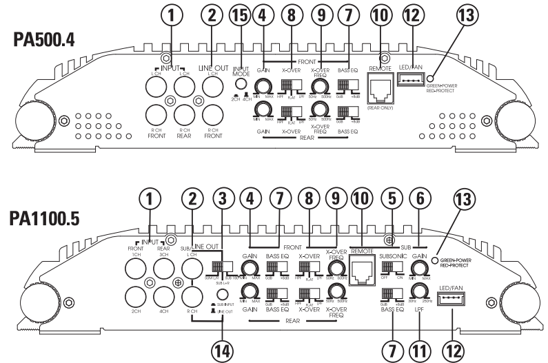
FIGURE 1b—«REMOTE» (PA500.4/PA1100.5)
