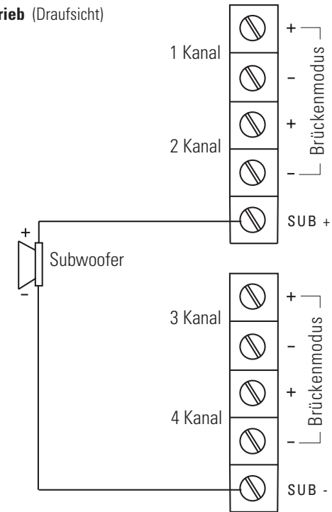
ABBILDUNG 4—LAUTSPRECHER-VERKABELUNGSDIAGRAMME (PA1100.5)
