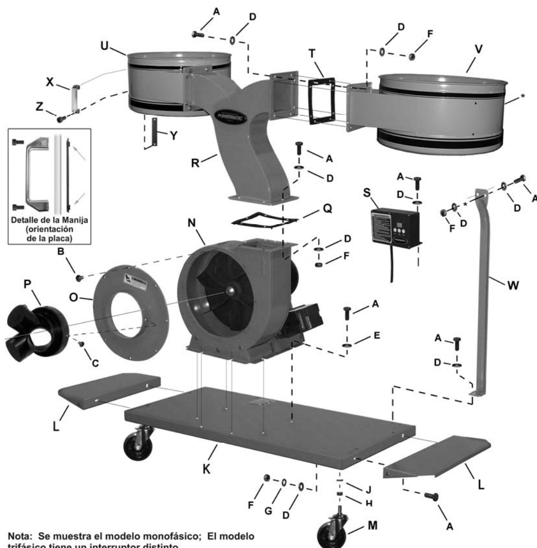
Figura 3: Montaje e Identificación de Partes
