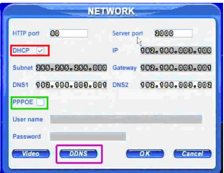
Image 6.2 Menu réseau
