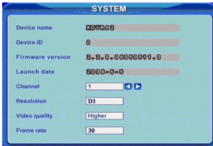
Image 5.4 Informations système
