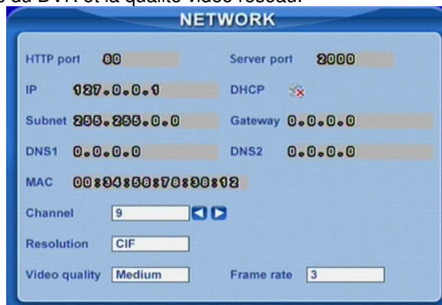
Image 5.5 Informations réseau
