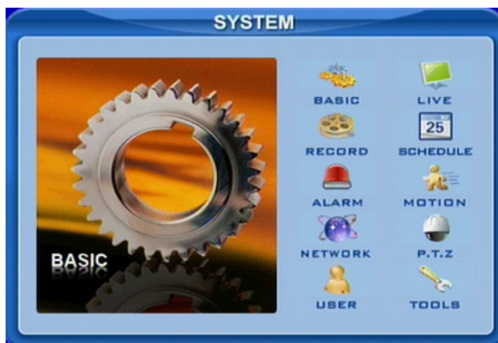
Image 4.3 Configuration système
