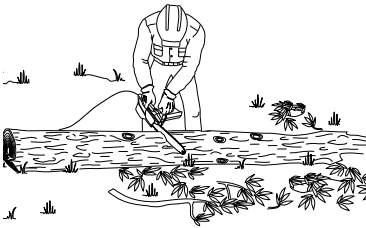
Figure 13 - Bucking Log With Entire Length On Ground Figura 13 - Trozado del tronco completamente apoyado en el suelo Figure 13 - Tronçonnage d'une bille qui repose entièrement au sol
