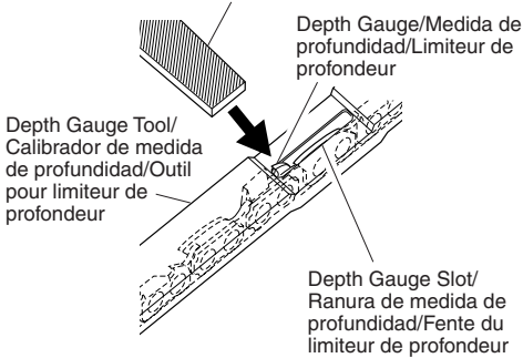
Figure 21 - Depth Gauge Tool On Chain Figura 21 - Calibrador de medida de profundidad en la cadena Figure 21 - Position de l'outil pour limiteur de profondeur sur la chaîne
