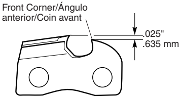
Figure 22 - Round Off Front Corner Of Depth Gauge Figura 22 - Redondeo del ángulo anterior de la medida de profundidad Figure 22 - Arrondir le coin avant du limiteur de profondeur
