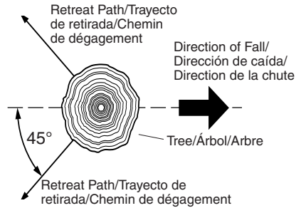
Figure 10 - Retreat Path From Tree Figura 10 - Trayecto de retirada de un árbol Figure 10 - Chemin de dégagement pour s'éloigner de l'arbre
