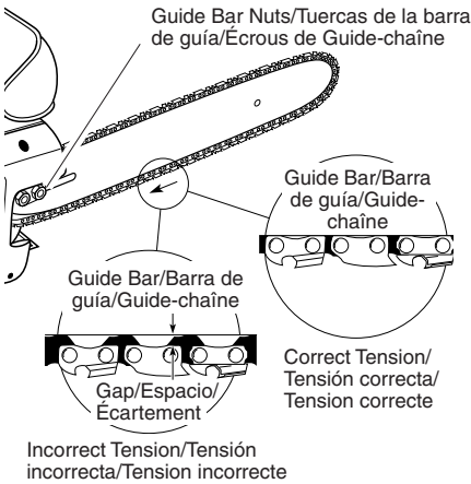
Figure 6 - Saw Chain Adjustment Figura 6 - Ajuste de la cadena serrada Figure 6 - Réglage de la chaîne
