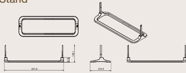
STN-L320PB (320PX)
