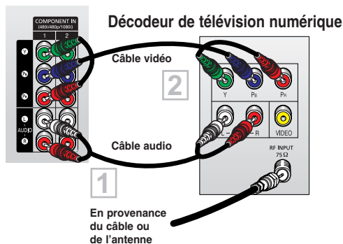
Panneau arrière du téléviseur
