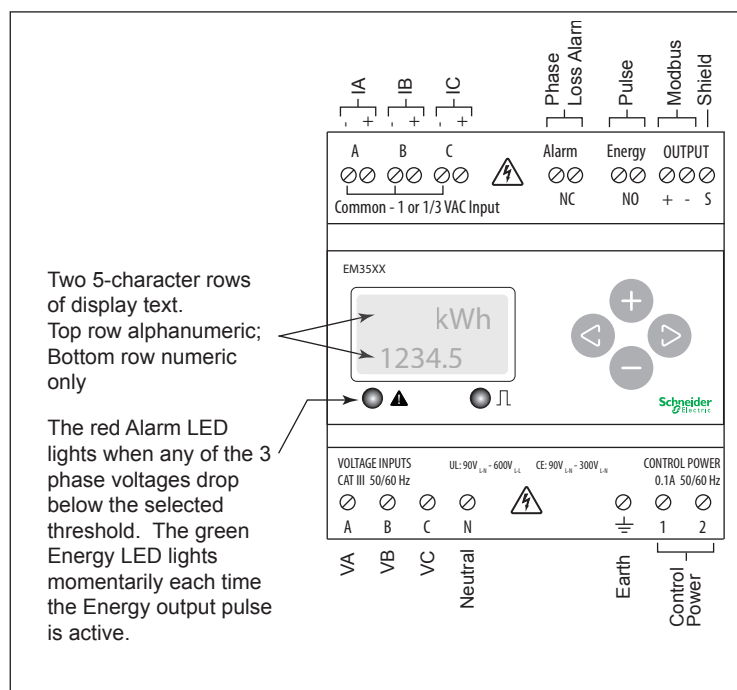
Figure 1 EM Series Meter
