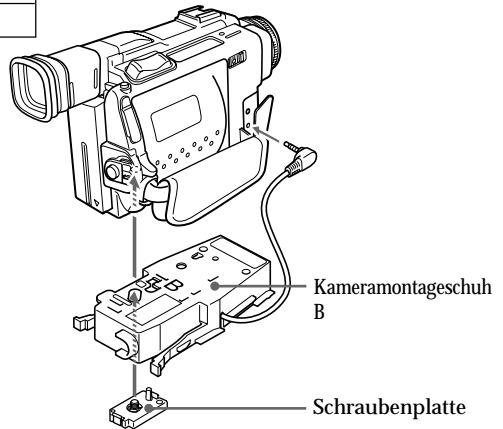
Montageposition der Schraubenplatte am Kameramontageschuh B
