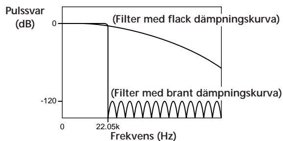
Jämförelse av skärningsegenskaper för filter med brant respektive flack dämpningskurva
