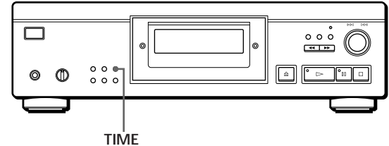
CDP-XA30ES
