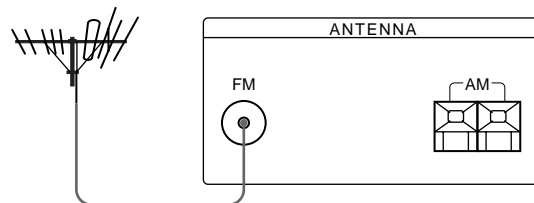
Conector IEC de tipo hembra
