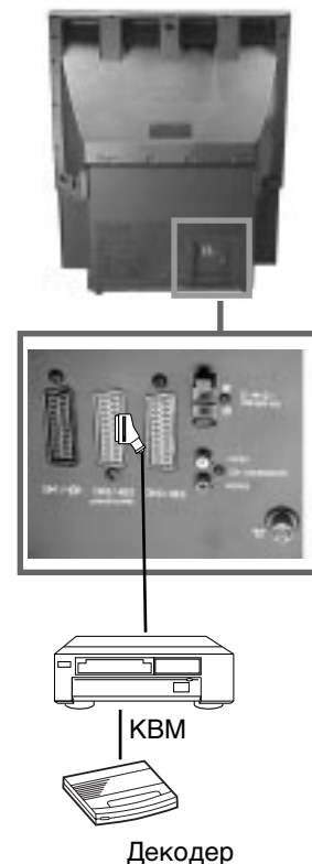
Задняя панель проекционного телевизора
