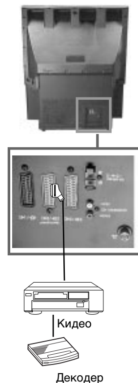
Задна страна на ретропроектора
