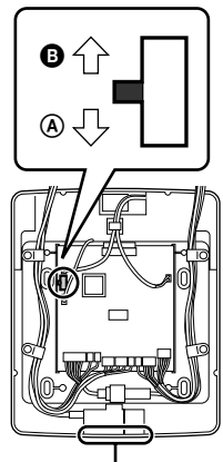
Récepteur de la télécommande carte
