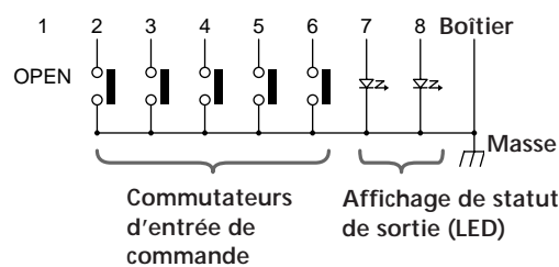
Schéma de connexion (MODE 1)
