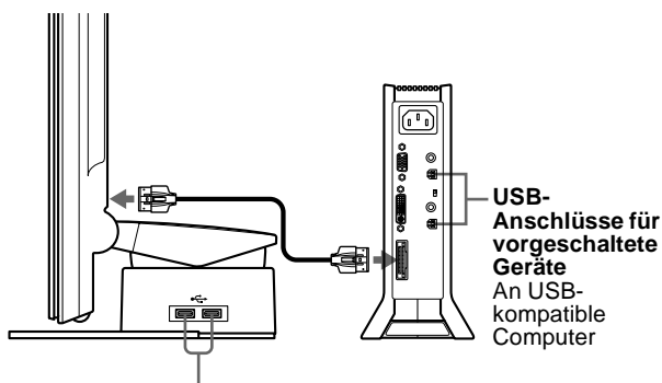
USB-Anschlüsse für nachgeschaltete Geräte An USB-kompatible Peripheriegeräte
