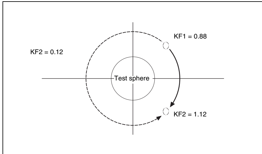
Keyframe trajectory
