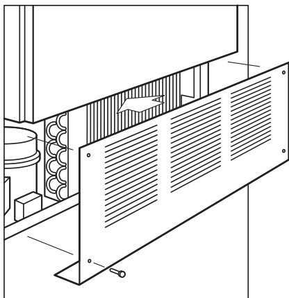
Position des Kondensators
