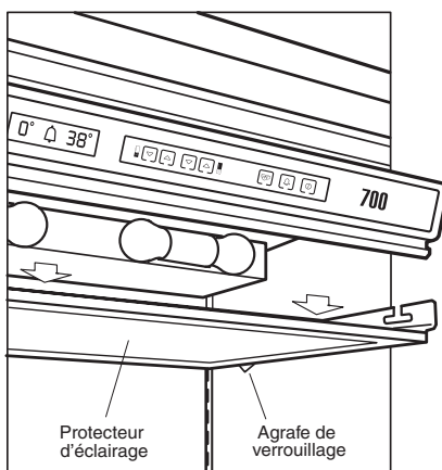
Emplacement de l'ampoule de la section supérieure
