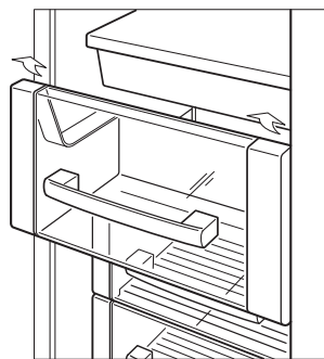
Rimozione secchiello ghiaccio—modelli ICBB1-36S, ICBB1-42S e ICBB1-48S
