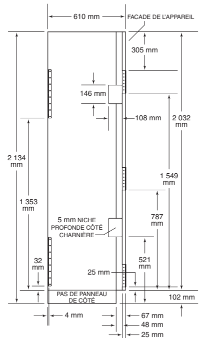
Spécifications concernant les panneaux de côté
