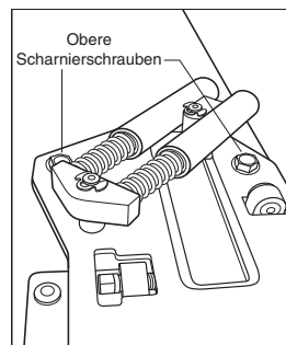
Türeinrichtung – obere Scharnierschraube
