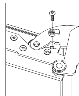
Fermaporta da 90 gradi
