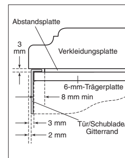
Verkleidungsplatte – Profilsicht
