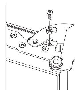
Türanschlag von 90 Grad
