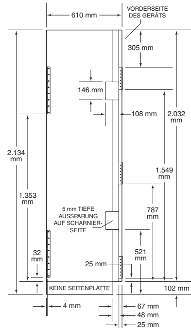
Technische Daten zu Seitenplatten
