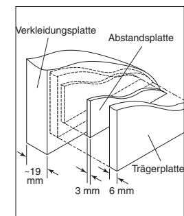
Verkleidungsplatte – Gruppe aus drei Platten
