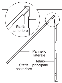
Attacco pannello laterale— vista superiore
