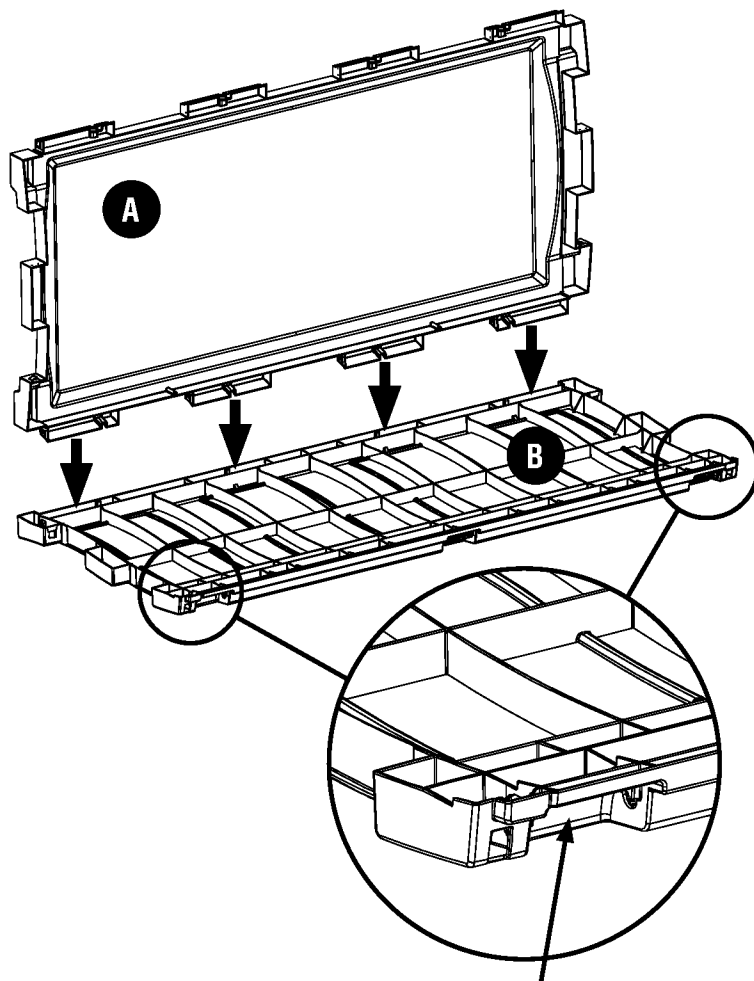
lid hinge receptacle logement de charnière de couvercle receptáculo de bisagra de tapa
