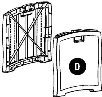
DBW7300 - #0102152B9 DBW9200 - #0102157B9 Side Côté Lateral x2
