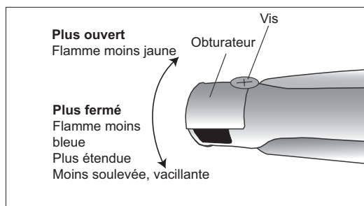
FIG. 15 Réglage de l'obturateur d'air (au besoin)
