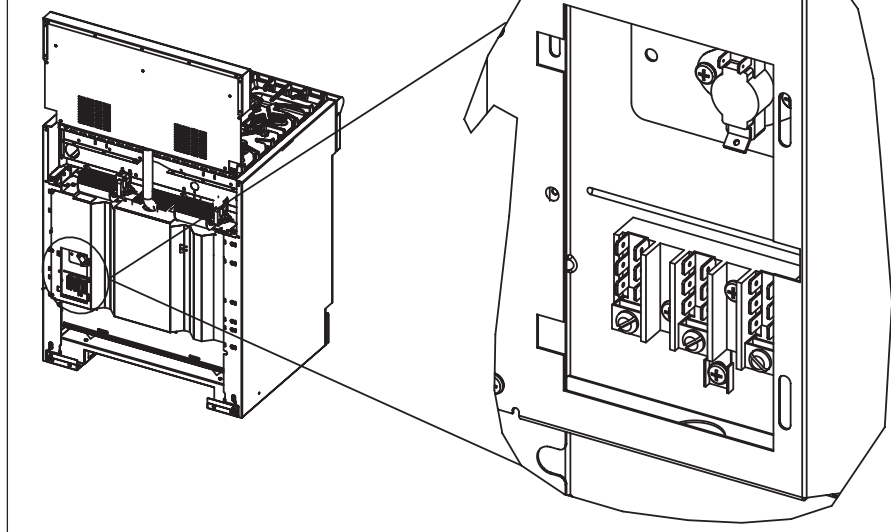
FIG. 8 - Emplacement de la boîte de jonction pour cuisinières à combustion jumelée
