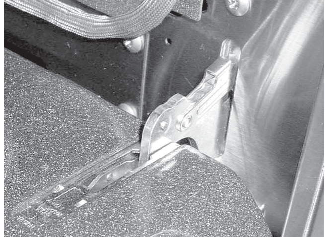
Photo B. Charnière en position fermée
