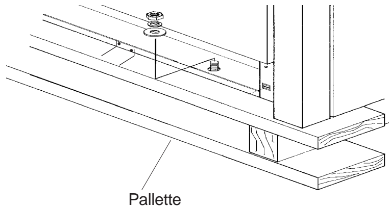
FIG. 4 – Retrait des quatre boulons avant installés pour l'expédition
