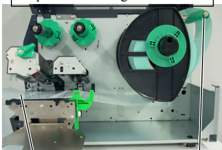
Guide Shaft
