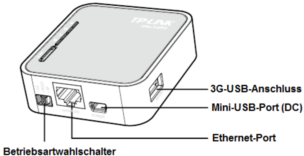
Bild 1-2 Geräteseitenansicht
