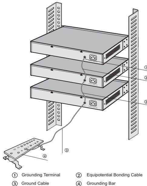
Figure 3-3 Equipotential Bonding
