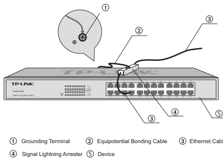
Figure 3-4 Equipotential Bonding
